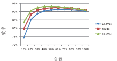
RSD-300C-48
