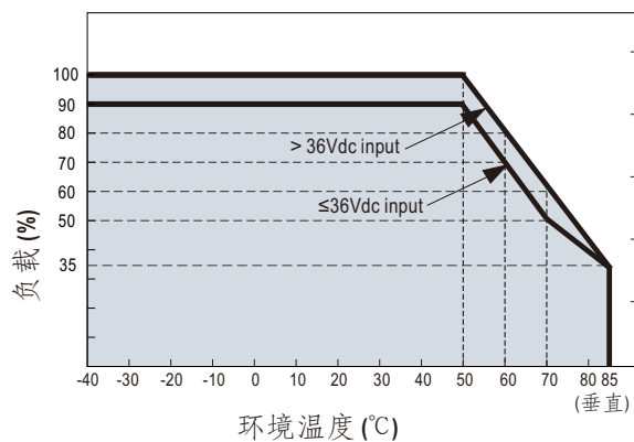
DDR-60L-5
