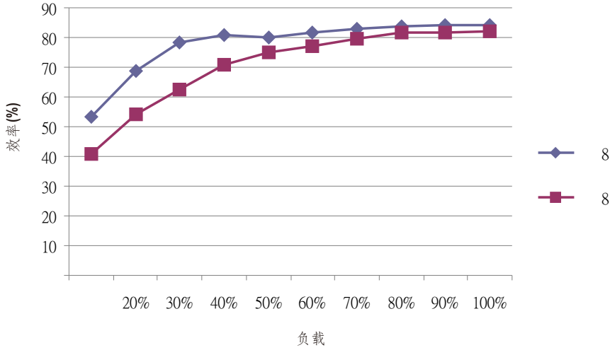
■ 效率vs负载(APC-12-350)
